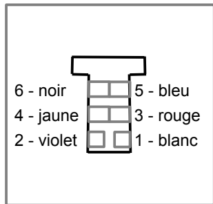
Socle « PTT » femelle Vu de dessus
